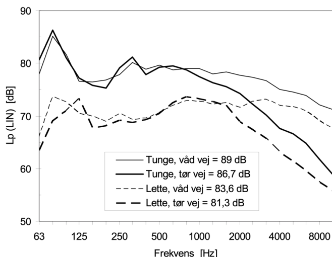
Figur 6. Exempel på bullerspektrum från lätta och tunga fordon på en motorväg med tät asfaltbetong (ABT), 110 km/h [28].
