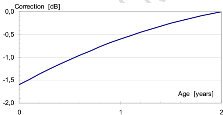
Figur 7. Ålderskorrektion för DAC- och SMA-vägytor. Korrektionen är 0 dB för vägytor äldre än 2 år [3].
